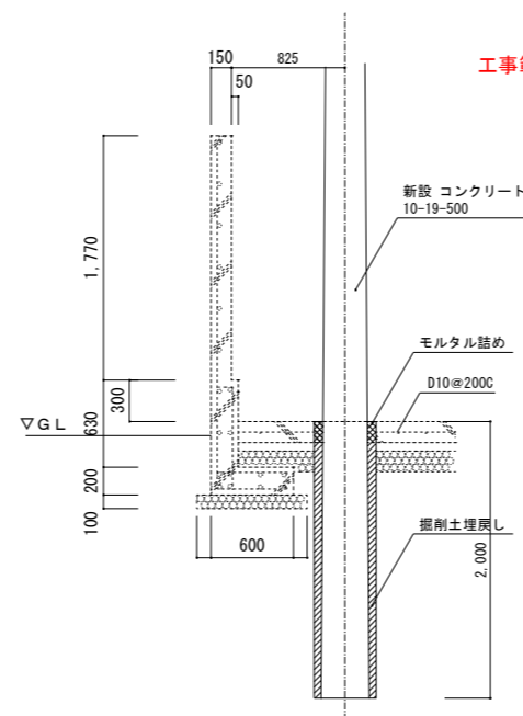
① 既存遮音壁+新設コンクリート柱 1/30
